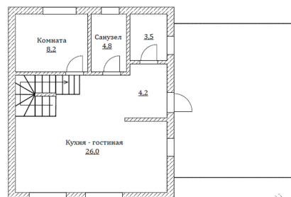
1 этаж
