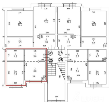
1- ЭТАЖ H=2.65
